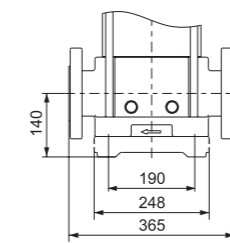
DIN FLANGE(LVR)/F
