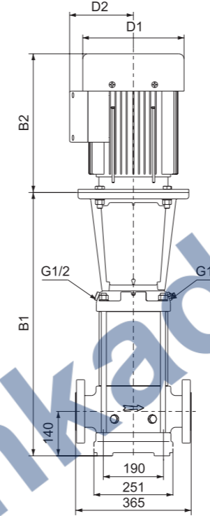
DIN FLANGE(LVS)/F
